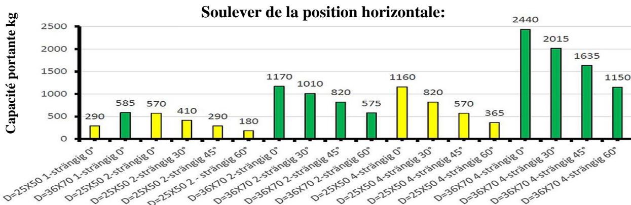
Chart 3: angle entre l'axe de la douille fileté et la direction de la fibre de bois 90° (Plus informations: www.rampa.com )
