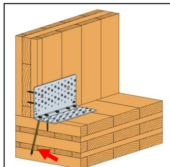
Typ AB: Vissage incliné dans l'angle
